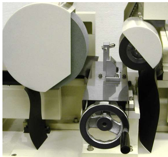
砥石車・調整車ツルーイング装置を装着したところ
