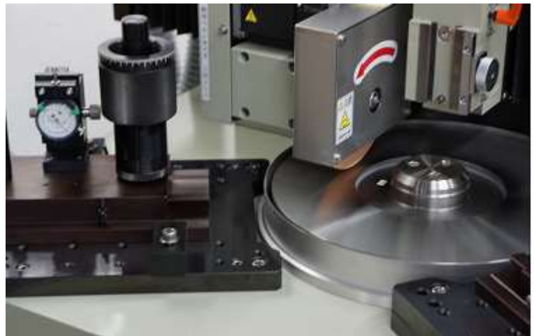
研削砥石によるスカイフ上面の修正
