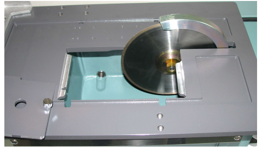
ブレード交換用フタを開けたところ TS-200PS2
