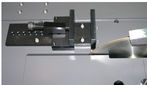
専用バイス取付例 TS-200PS2
