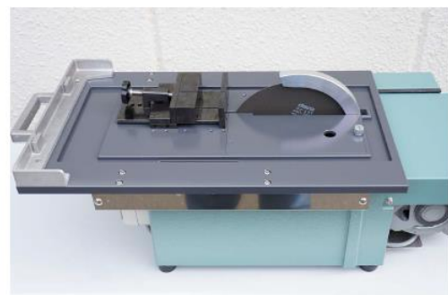
専用バイスダブルタイプを装着したところ
