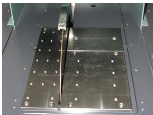
補助テーブル取付例（別売）
