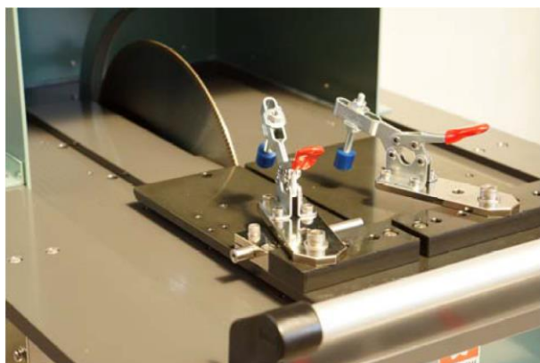
トルクランプ取付例
