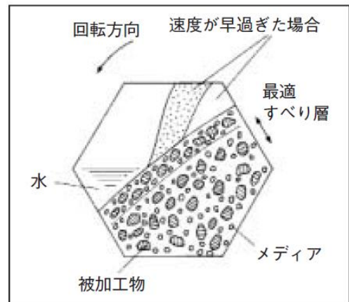
バレル内部の運動解析
